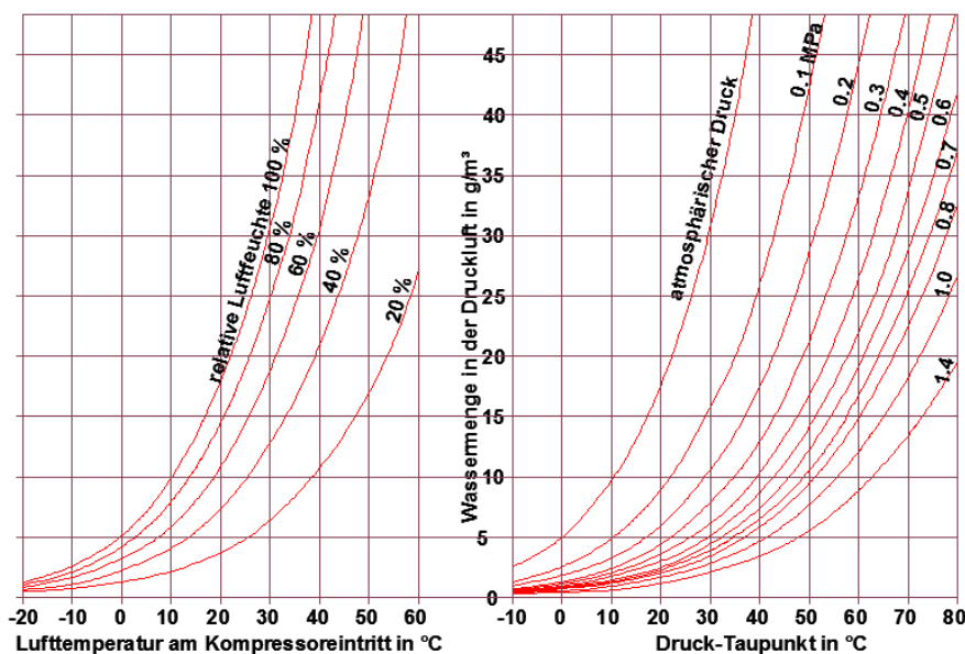
Abb. 1 Anfallende Kondensatmenge
